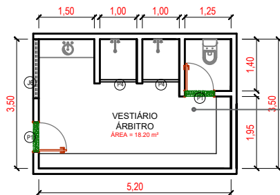
PLANTA BAIXA | VESTIÁRIO ESCALA 1/100
